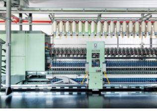
Şek. 1: Beste, ROBOspin robotuyla donatılmış tam elektronik ring iplik makinası G 38 ile en yüksek kalitede iplikler üretir.
